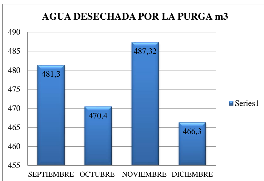
Gráfico 28: Cantidad de agua desechada por la purga.
