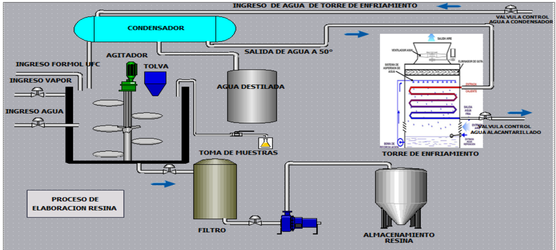
Gráfico 25: Proceso de elaboración resina.
