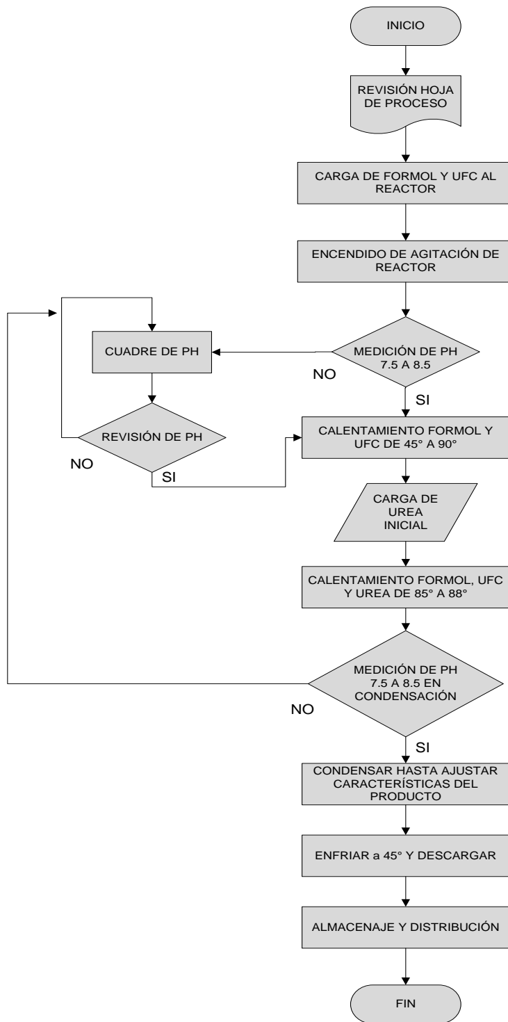
Gráfico 22: Proceso elaboración resina.
