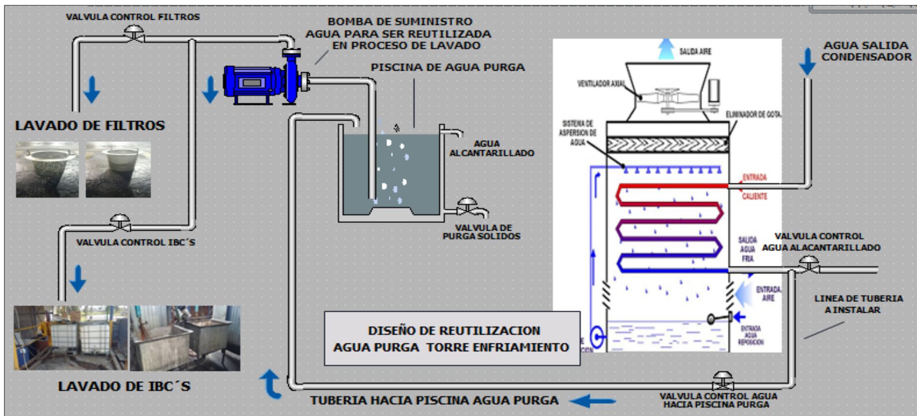
Gráfico 38: Diseño de propuesta uso agua purga.
