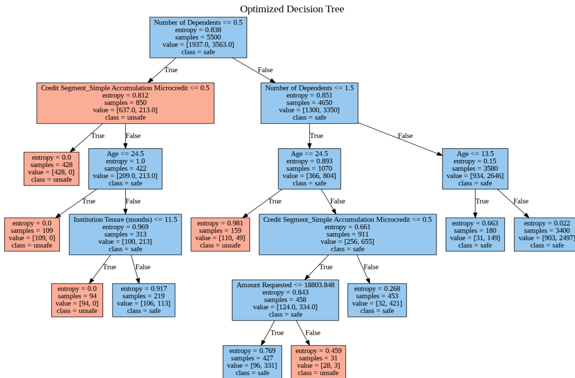
Diagrama de árbol de decisión, resaltando las reglas de clasificación
