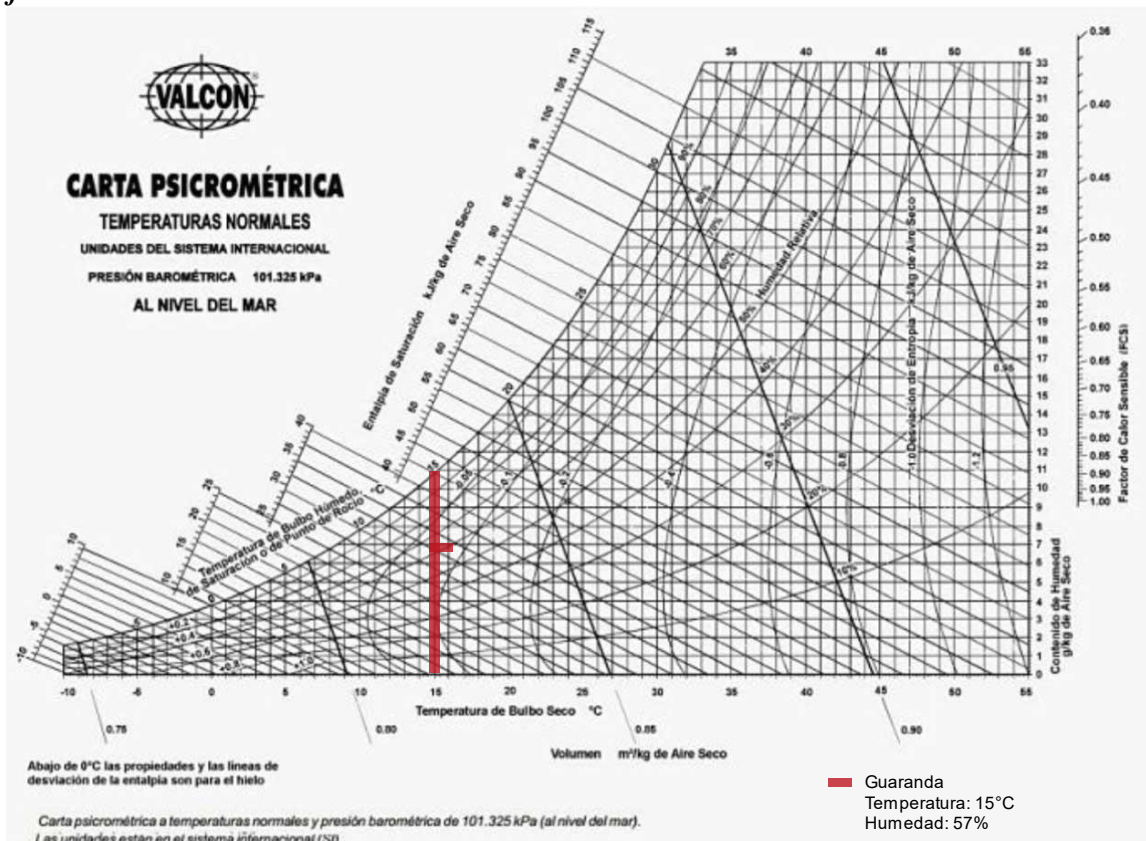
Gráfico 33. Carta Psicrométrica
